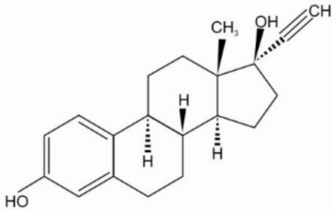
Ethinyl Estradiol C_{20}H_{24}O_2 MW: 296.4
