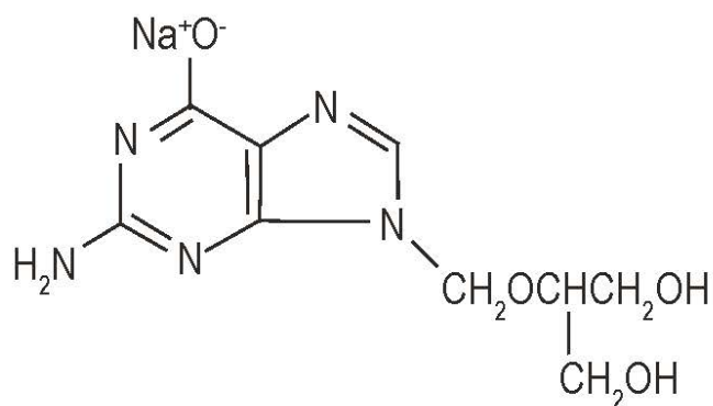
ganciclovir sodium C_9H_{12}N_5NaO_4 M.W.=277.22
