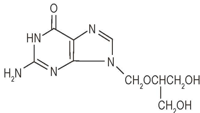
ganciclovir C_9H_{13}N_5O_4 M.W.=255.23
