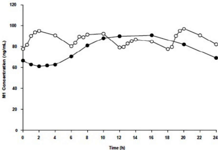
a. Tramadol
