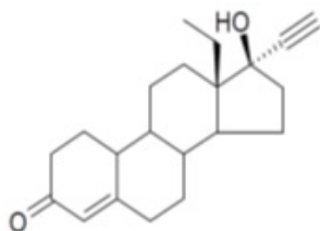
Levonorgestrel C 21 H 28 O 2 M.W. 312.5
