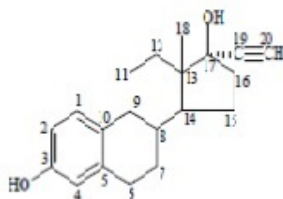
Ethinyl Estradiol C 20 H 24 O 2 M.W. 296.41
