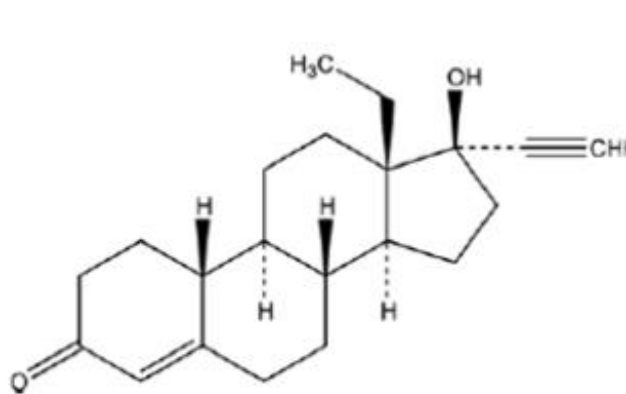
Levonorgestrel C 21 H 28 O 2 M.W. 312.45
