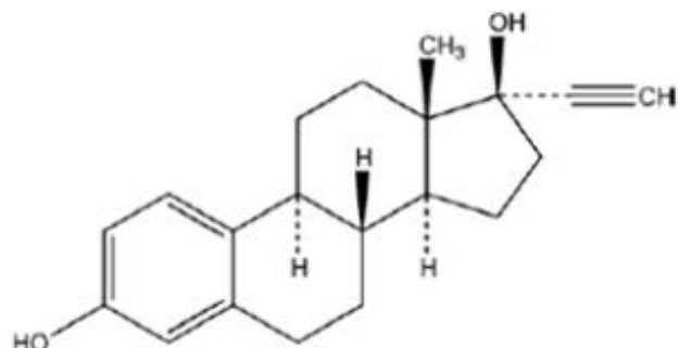
Ethinyl Estradiol C 20 H 24 O 2 M.W. 296.40
