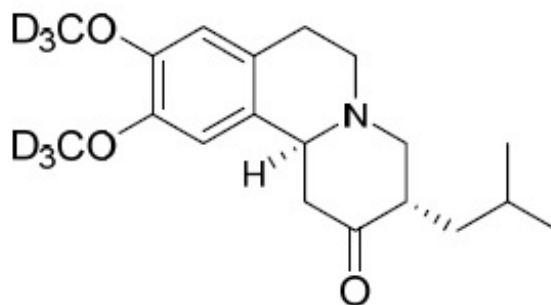
SS - Deutetrabenazine
