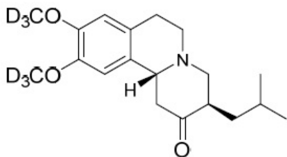
RR - Deutetrabenazine
