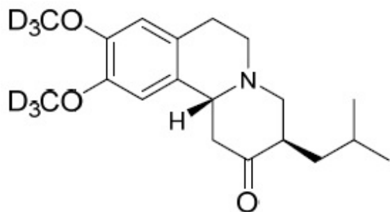
RR - Deutetrabenazine
