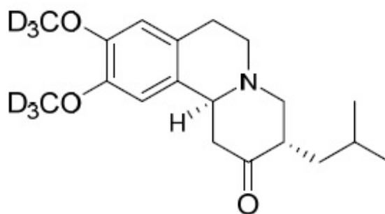
SS - Deutetrabenazine
