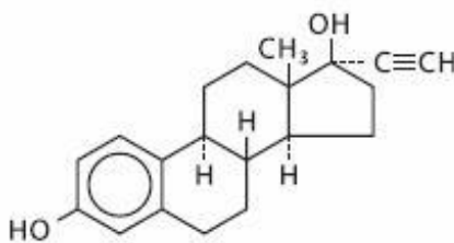
Ethinyl Estradiol
