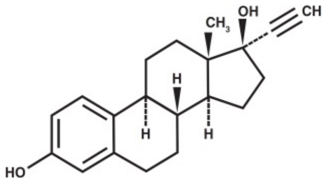
Ethinyl Estradiol C_{20}H_{24}O_2 MW: 296.4
