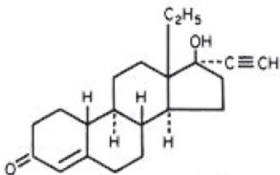
Levonorgestrel C_{21}H_{28}O_2 M.W. 312.45
