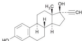
Ethinyl estradiol
