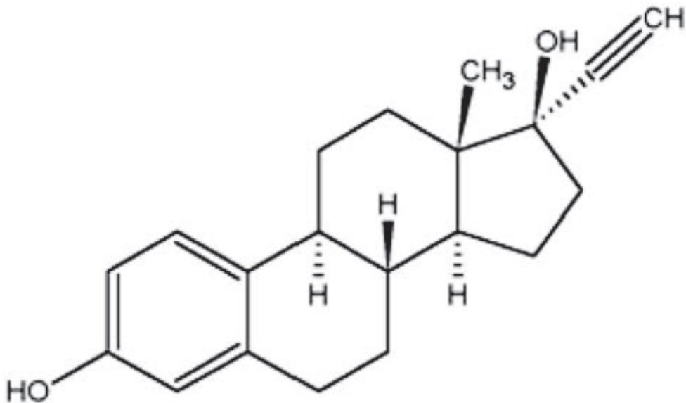
Ethinyl Estradiol C_{20}H_{24}O_2 MW: 296.4
