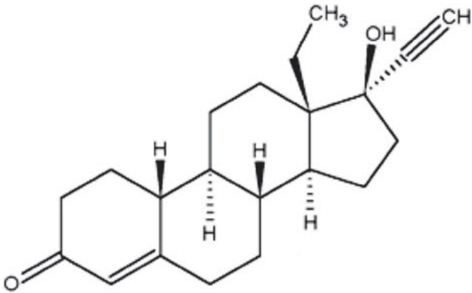
Levonorgestrel C_{21}H_{28}O_2 MW: 312.4
